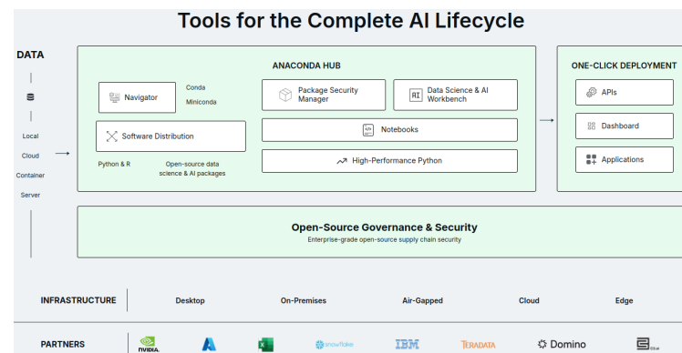
图 3: Anaconda 面向 AI 生命周期的工具集
