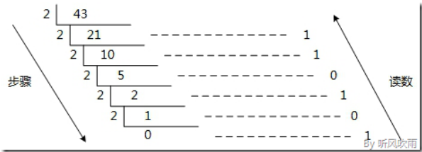
图 4: 除 n 取余法 (43→101011)
