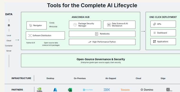
图 3: Anaconda 面向AI生命周期的工具集
