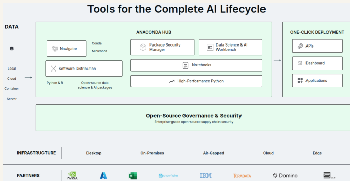
图 3: Anaconda 面向AI生命周期的工具集
